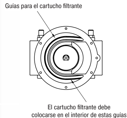
fig. a: Cuerpo DN 15 ÷ DN 50 sin tapa inferior
